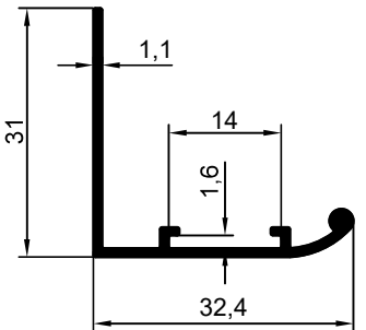
1960 0.225 kg/m
