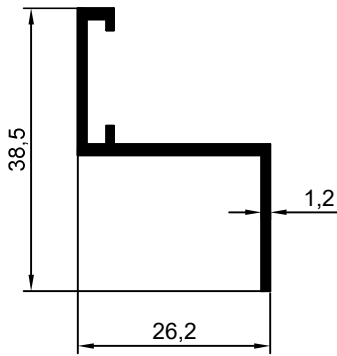
1949 0.252 kg/m
