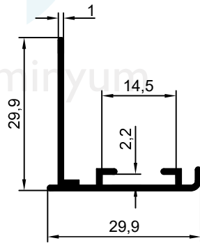
1920 0.206 kg/m
