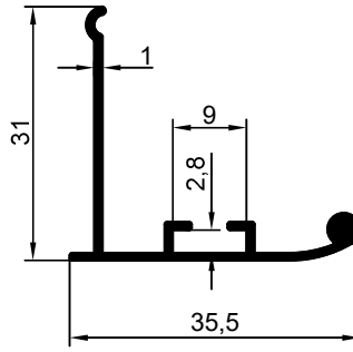
1930 0.232 kg/m
