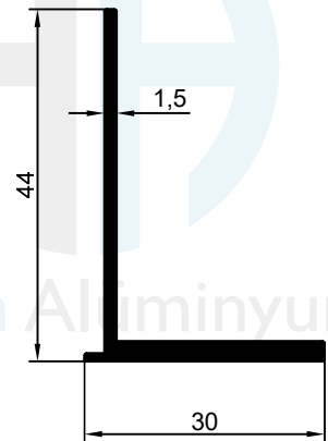
2503 0.361 kg/m
