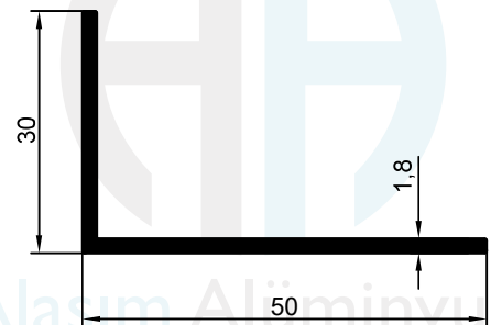
2116 0.382 kg/m
