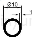
2094 0.076 kg/m
