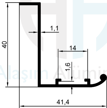
2152 0.270 kg/m
