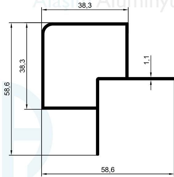
3004 0.558 kg/m
