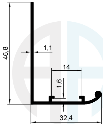
1961 0.271 kg/m
