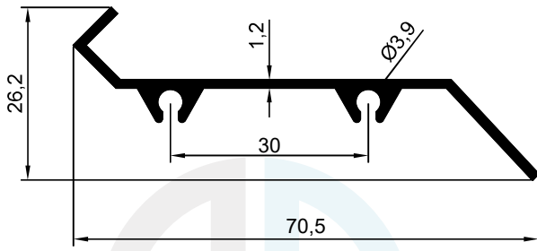
1934 0.400 kg/m
