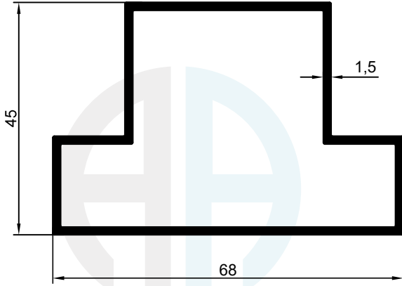
3011 0.894 kg/m
