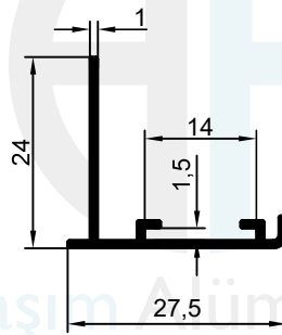
2504 0.168 kg/m
