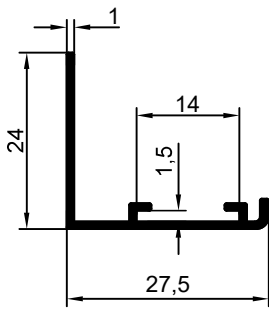
2505 0.170 kg/m
