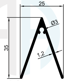
2155 0.252 kg/m
