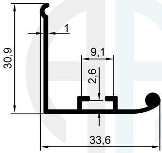
1931 0.227 kg/m
