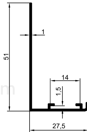
2506 0.241 kg/m
