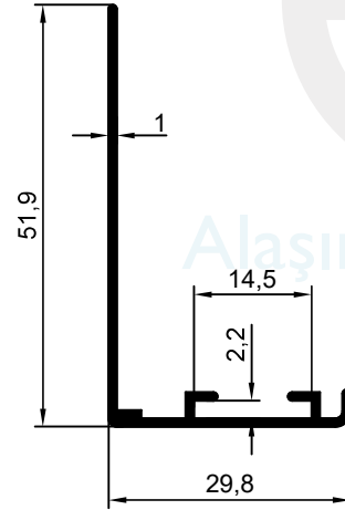
1915 0.266 kg/m
