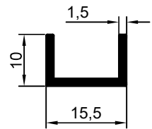
2117 0.133 kg/m
