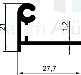
1928 0.244 kg/m
