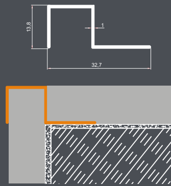
ALÜMİNYUM KARE KÖŞE FAYANS PROFİLİ Aluminum Square Corner Tile Profile
