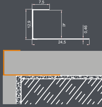
ALÜMİNYUM KARE DİŞ KÖŞE FAYANS PROFİLİ Aluminum Square Exterior Corner Tile Profile
