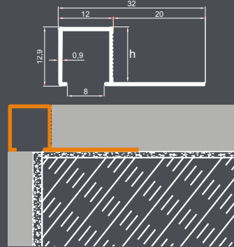
ALÜMİNYUM KARE KÖŞE FAYANS PROFİLİ Aluminum Square Corner Tile Profile
