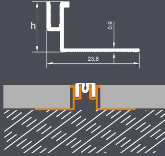
ALÜMİNYUM FAYANS GENLEŞME PROFİLİ Aluminum Tile Expansion Profile
