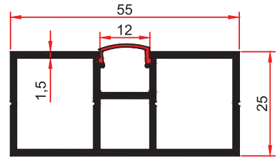
5542 0,802kg/m
