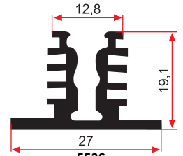
5536 0.430 kg/m
