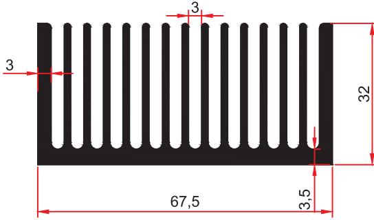
5531 2.627kg/m
