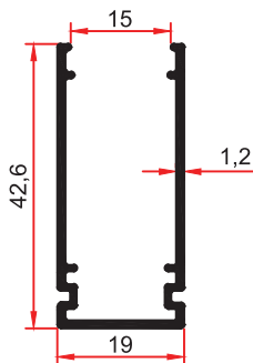
5544 0.363 Kg/m
