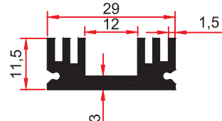
5528 0.476kg/m
