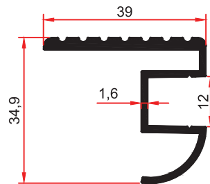
5546 0,566 kg/m
