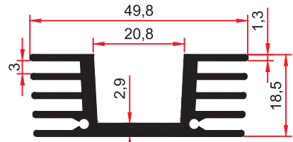
5532 0.848 kg/m
