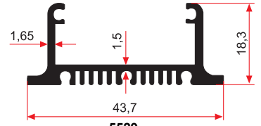
5529 0.488 kg/m
