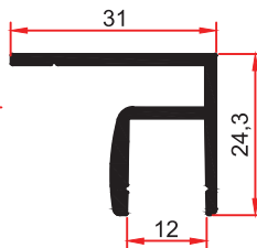
5545 0,389 kg/m
