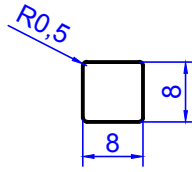
2258 0.173 kg/m
