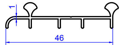
2092 0.276 kg/m
