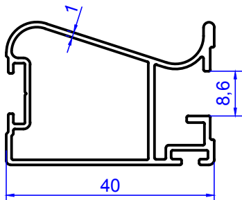
2056 0.472 kg/m
