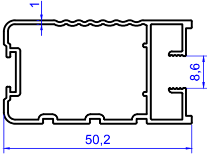
2058 0.558 kg/m
