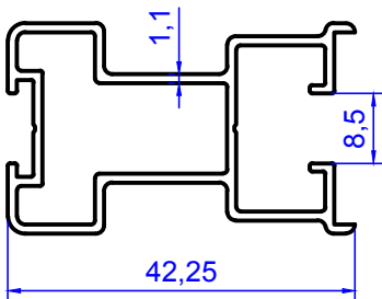
2048 0.496 kg/m
