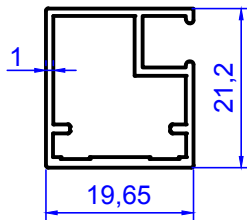
2238 0.263 kg/m
