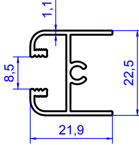
2035 0.279 kg/m
