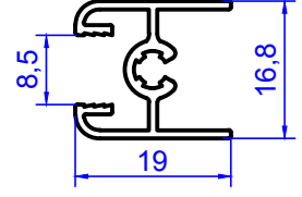
2033 0.211 kg/m
