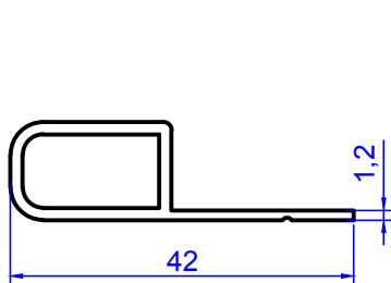
2141 0.293 kg/m
