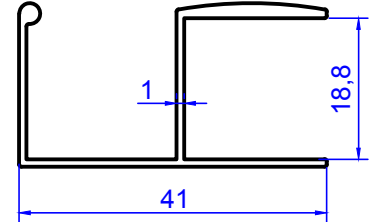
2149 0.363 kg/m
