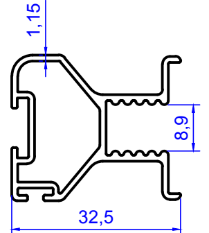
2065 0.458 kg/m
