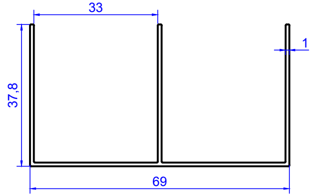
2104 0.545 kg/m
