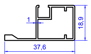
2224 0.309 kg/m
