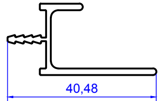
2128 0.318 kg/m
