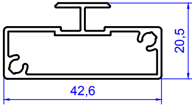
2228 0.481 kg/m
