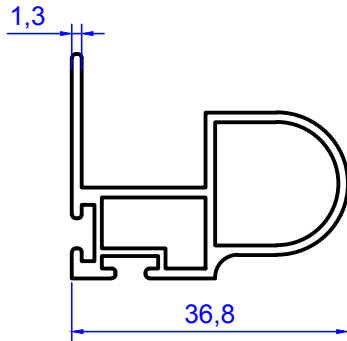
2135 0.493 kg/m
