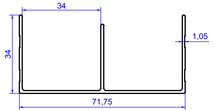
2106 0.553 kg/m
