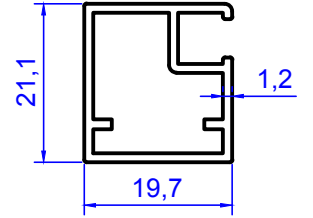
2221 0.295 kg/m
