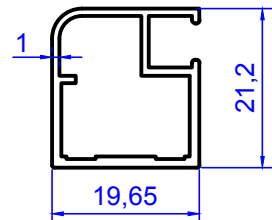
2239 0.268 kg/m
