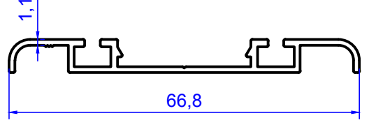
2083 0.325 kg/m
