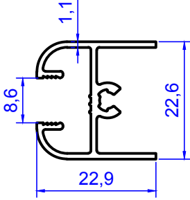
2034 0.287 kg/m
