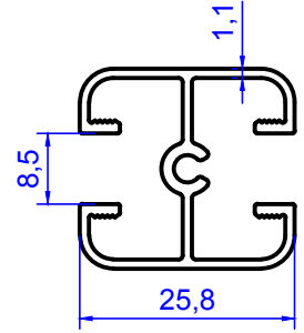
2021 0.370 kg/m
