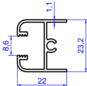
2029 0.280 kg/m
