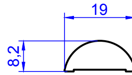
2261 0.303 kg/m
