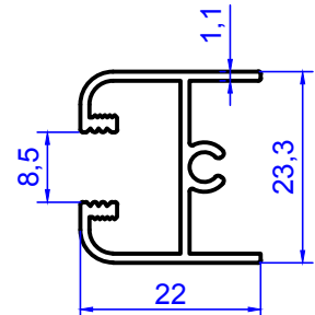
2030 0.285 kg/m
