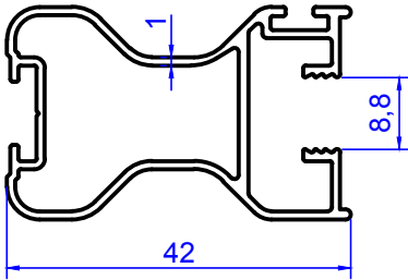
2054 0.485 kg/m
