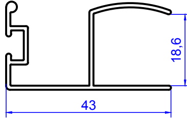
2148 0.360 kg/m
