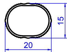
2250 0.119 kg/m
