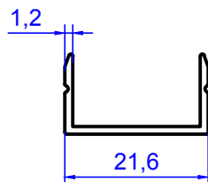
2175 0.130 kg/m
