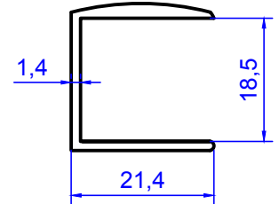
2170 0.252 kg/m
