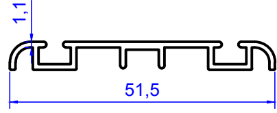
2085 0.271 kg/m
