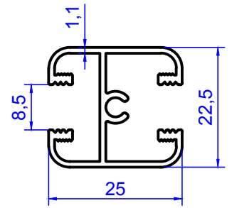
2027 0.358 kg/m
