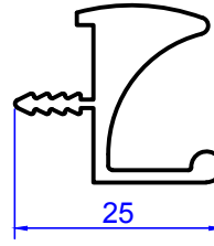
2124 0.429 kg/m
