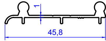
2089 0.293 kg/m
