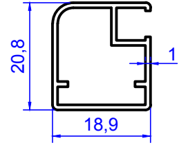
2218 0.230 kg/m
