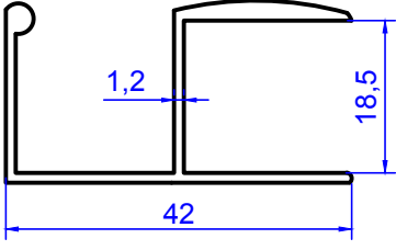
2144 0.393 kg/m
