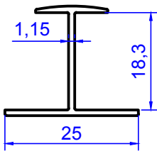
2162 0.168 kg/m
