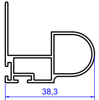
2137 0.452 kg/m
