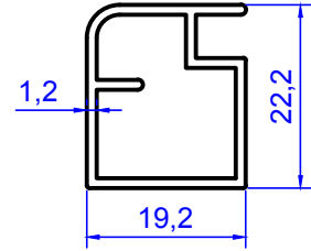
2230 0.285 kg/m
