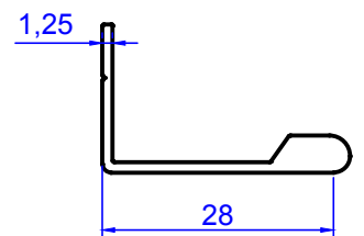
2143 0.225 kg/m
