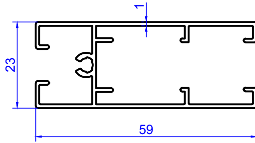
2007 0.545 kg/m
